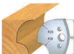
Par de cuchillas: 690.549 Par contracuchillas: 691.549
