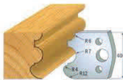
Par de cuchillas 690.088 Par contracuchillas 691.088
