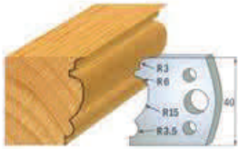
Par de cuchillas 690.104 Par contracuchillas 691.104
