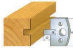
Par de cuchillas 690.094 Par contracuchillas 691.094
