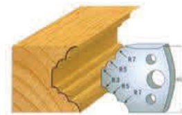
Par de cuchillas 690.021 Par contracuchillas 691.021
