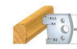
Par de cuchillas 690.130 Par contracuchillas 691.130
