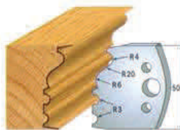
Par de cuchillas 690.513 Par contracuchillas 691.513
