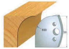
Par de cuchillas 690.568 Par contracuchillas 691.568
