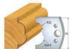
Par de cuchillas 690.519 Par contracuchillas 691.519
