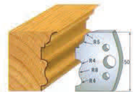
Par de cuchillas 690.515 Par contracuchillas 691.515
