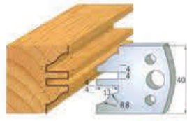
Par de cuchillas 690.097 Par contracuchillas 691.097
