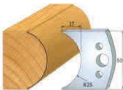
Par de cuchillas: 690.546 Par contracuchillas: 691.546
