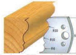
Par de cuchillas 690.506 Par contracuchillas 691.506
