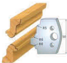
Par de cuchillas: 690.542 Par contracuchillas: 691.542
