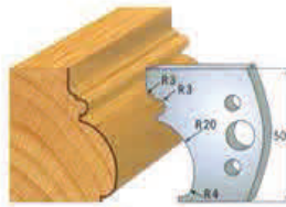
Par de cuchillas 690.501 Par contracuchillas 691.501
