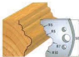
Par de cuchillas 690.508 Par contracuchillas 691.508
