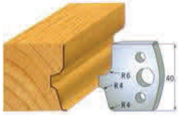
Par de cuchillas 690.041 Par contracuchillas 691.041
