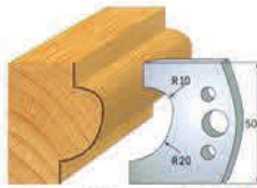
Par de cuchillas 690.504 Par contracuchillas 691.504
