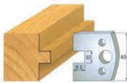
Par de cuchillas 690.092 Par contracuchillas 691.092
