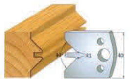
Par de cuchillas 690.071 Par contracuchillas 691.071
