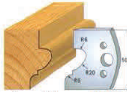
Par de cuchillas 690.505 Par contracuchillas 691.505
