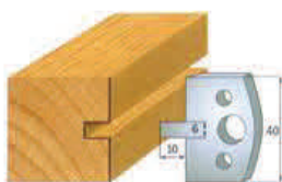
Par de cuchillas 690.016 Par contracuchillas 691.016
