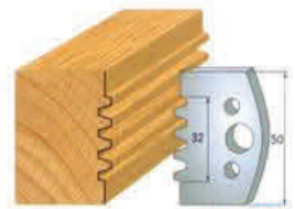
Par de cuchillas 690.576 Par contracuchillas 691.576
