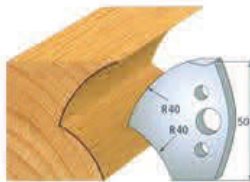
Par de cuchillas: 690.550 Par contracuchillas: 691.550
