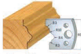
Par de cuchillas 690.102 Par contracuchillas 691.102
