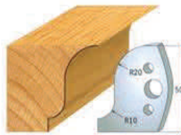
Par de cuchillas 690.570 Par contracuchillas 691.570
