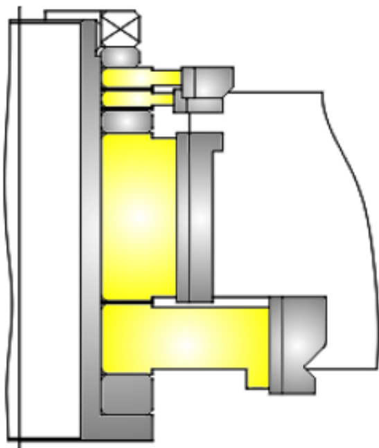
CONJUNTO RETESTAR CORREDERA TRAVESAÑO PERFILES 6040
